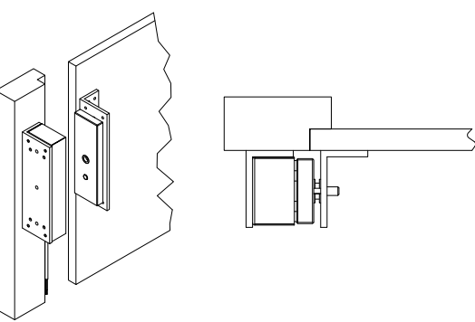
Sliding door
